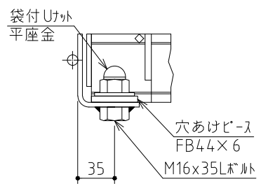
ボルト固定部詳細
